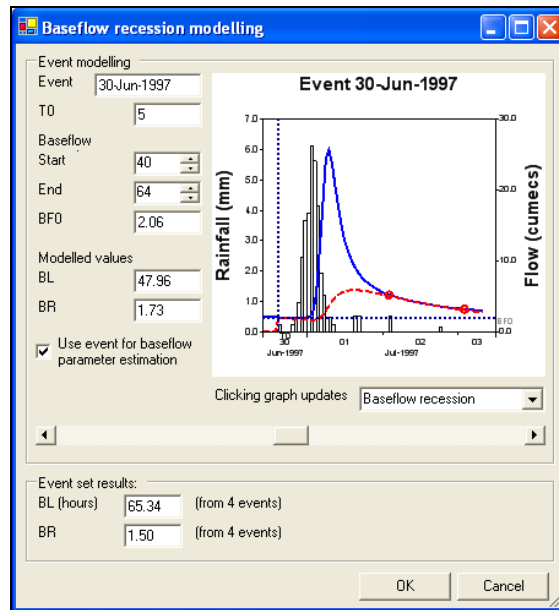
Figure 3.7 Baseflow parameter estimation module
